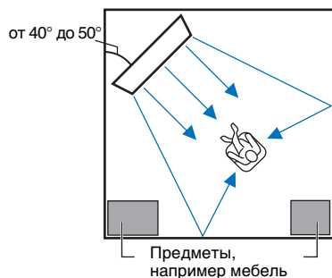
Угловая установка: вид сверху
