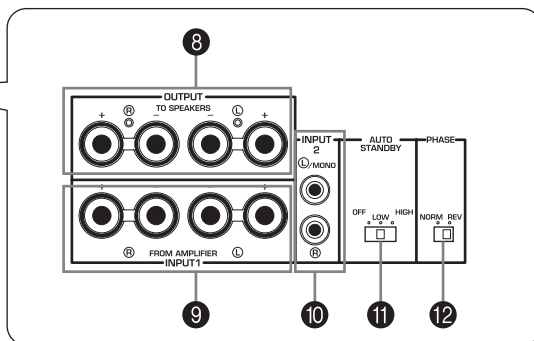
Задняя панель (общая модель)
